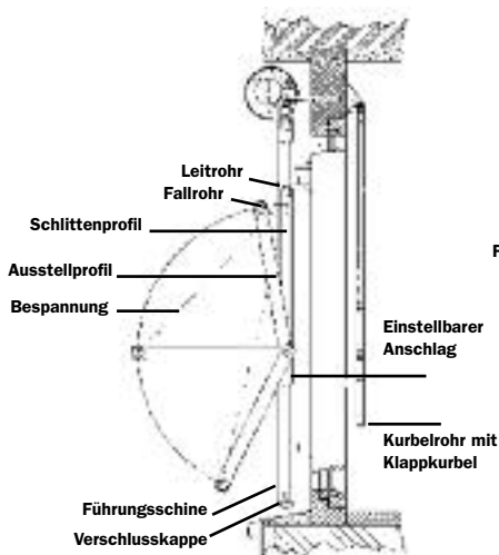
Markisolette im Seitenriss
