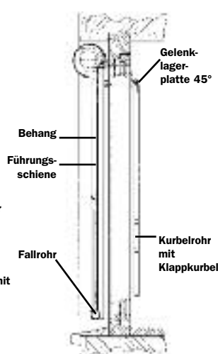
Außenrollo im Seitenriss
